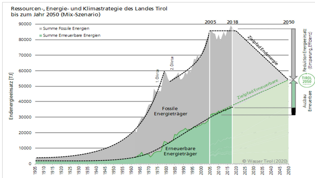
Abbildung 19: Energieeinsatz und erneuerbare Energien
