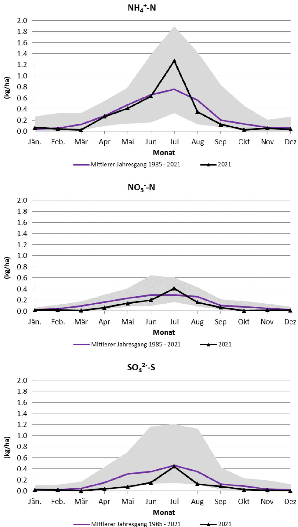
Abbildung 13: Darstellung der mittleren monatlichen Einträge in der Untersuchungsperiode 2021 im Vergleich zu den mittleren Jahresgängen an der Messstelle in Innervillgraten . Die grau hinterlegte Fläche stellt die Schwankungsbreite der bisher bestimmten Monatswerte dar. Weitere Angaben im Text.
