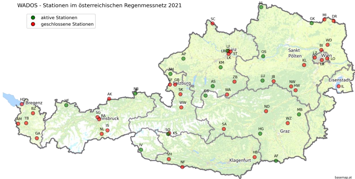
Abbildung 2: Lage der WADOS - Stationen im österreichischen Niederschlagsmessnetz für das Niederschlagsjahr 2021
