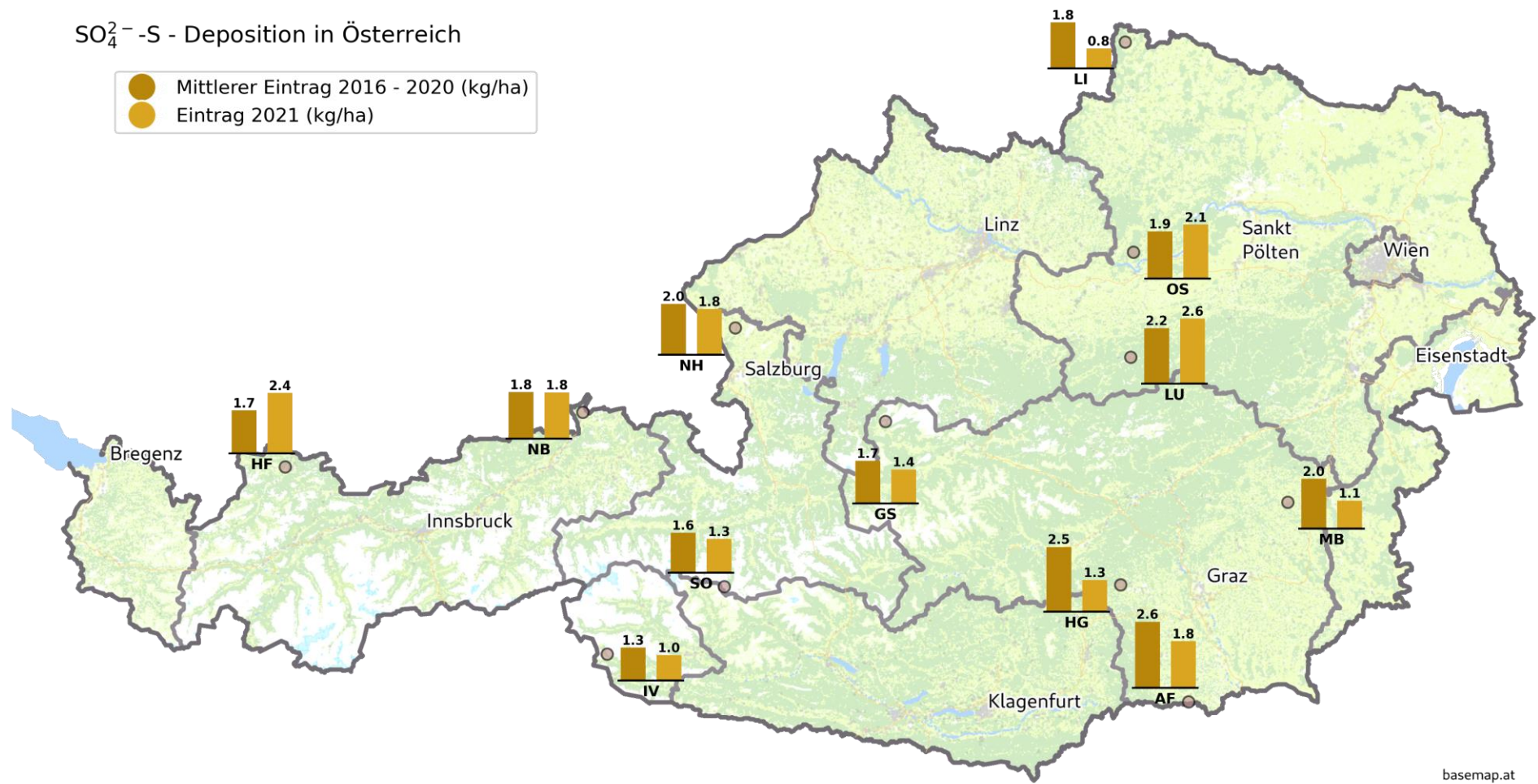
Abbildung 33: Räumliche Verteilung der SO 4 2- -S-Jahreseinträge für den Zeitraum Jänner 2021 bis Dezember 2021 im Vergleich mit dem Mittelwert der letzten 5 Jahre.
