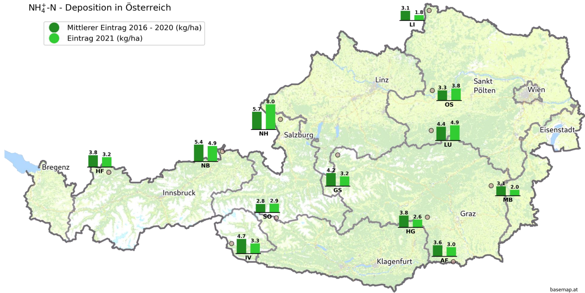
Abbildung 29: Räumliche Verteilung der NH 4 + -N-Jahreseinträge für den Zeitraum Jänner 2021 bis Dezember 2021 im Vergleich mit dem Mittelwert der letzten 5 Jahre.
