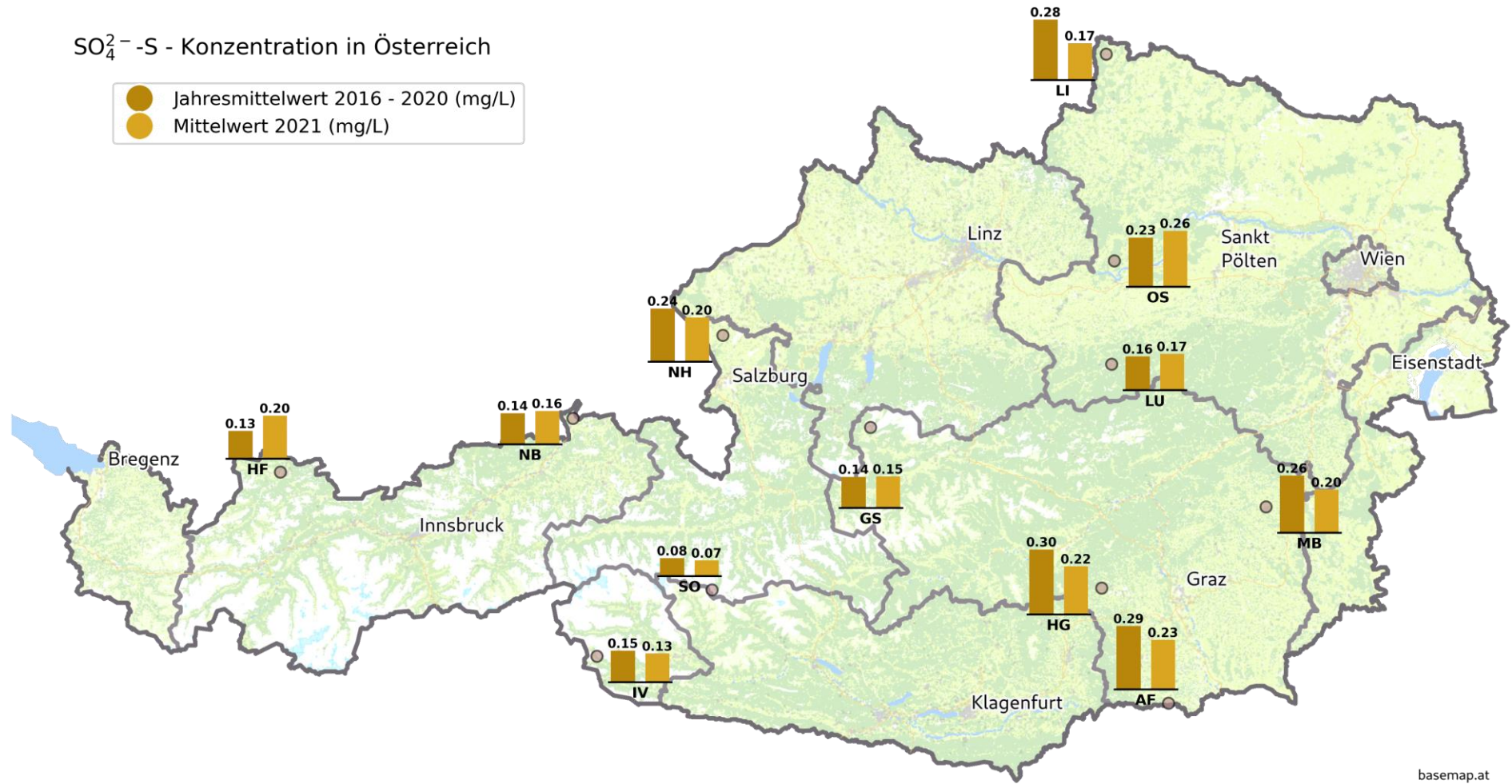
Abbildung 32: Räumliche Verteilung der mengengewichteten SO 4 2- -S-Jahreskonzentrationen für den Zeitraum Jänner 2021 bis Dezember 2021 im Vergleich mit dem Mittelwert der letzten 5 Jahre.
