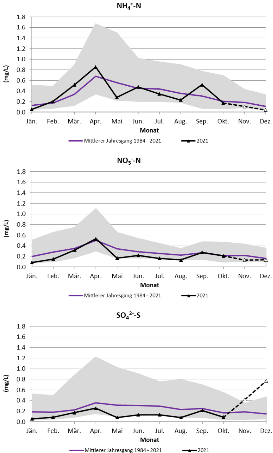
Abbildung. 8: Darstellung der mittleren monatlichen Konzentrationen in der Untersuchungsperiode 2021 im Vergleich zu den mittleren Jahresgängen an der Messstelle in Höfen . Die grau hinterlegte Fläche stellt die Schwankungsbreite der bisher bestimmten Monatswerte dar. Weitere Angaben im Text.
