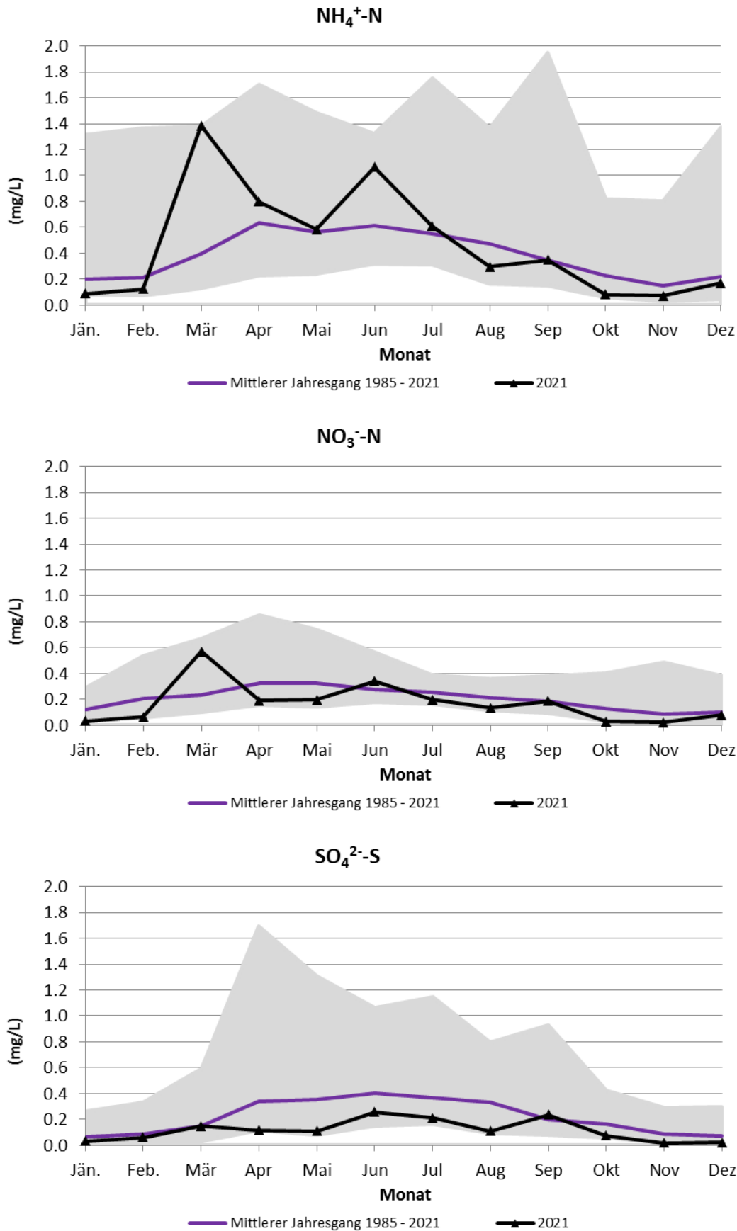
Abbildung. 12: Darstellung der mittleren monatlichen Konzentrationen in der Untersuchungsperiode 2021 im Vergleich zu den mittleren Jahresgängen an der Messstelle in Innervillgraten . Die grau hinterlegte Fläche stellt die Schwankungsbreite der bisher bestimmten Monatswerte dar. Weitere Angaben im Text.
