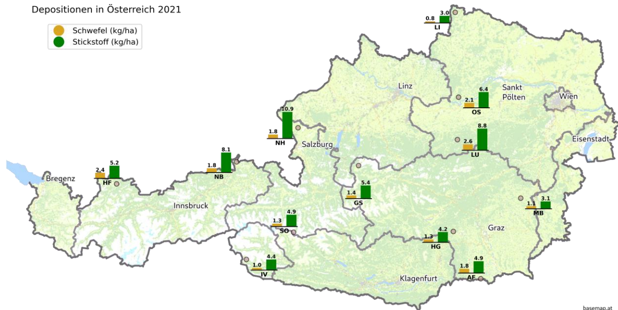
Abbildung 1: Schwefel- und Stickstoffdepositionen im Untersuchungszeitraum 2021.
