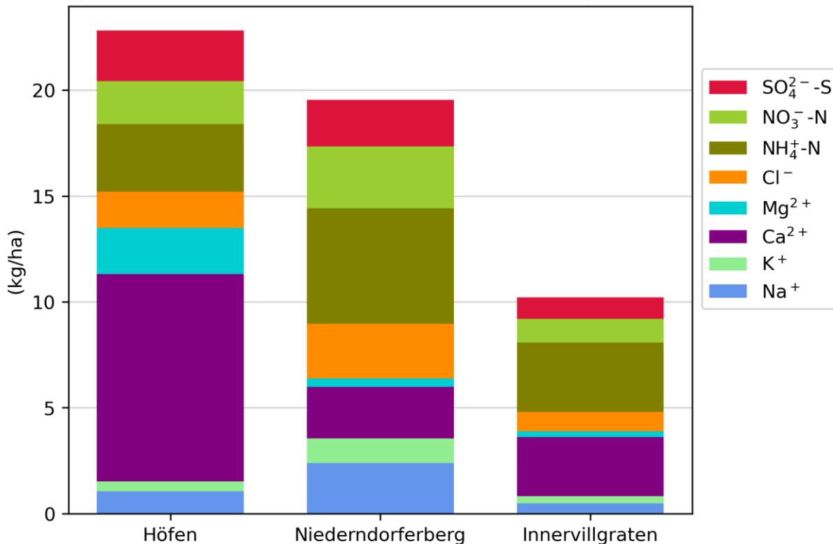
Deposition der einzelnen Ionen im Untersuchungsjahr 2021
