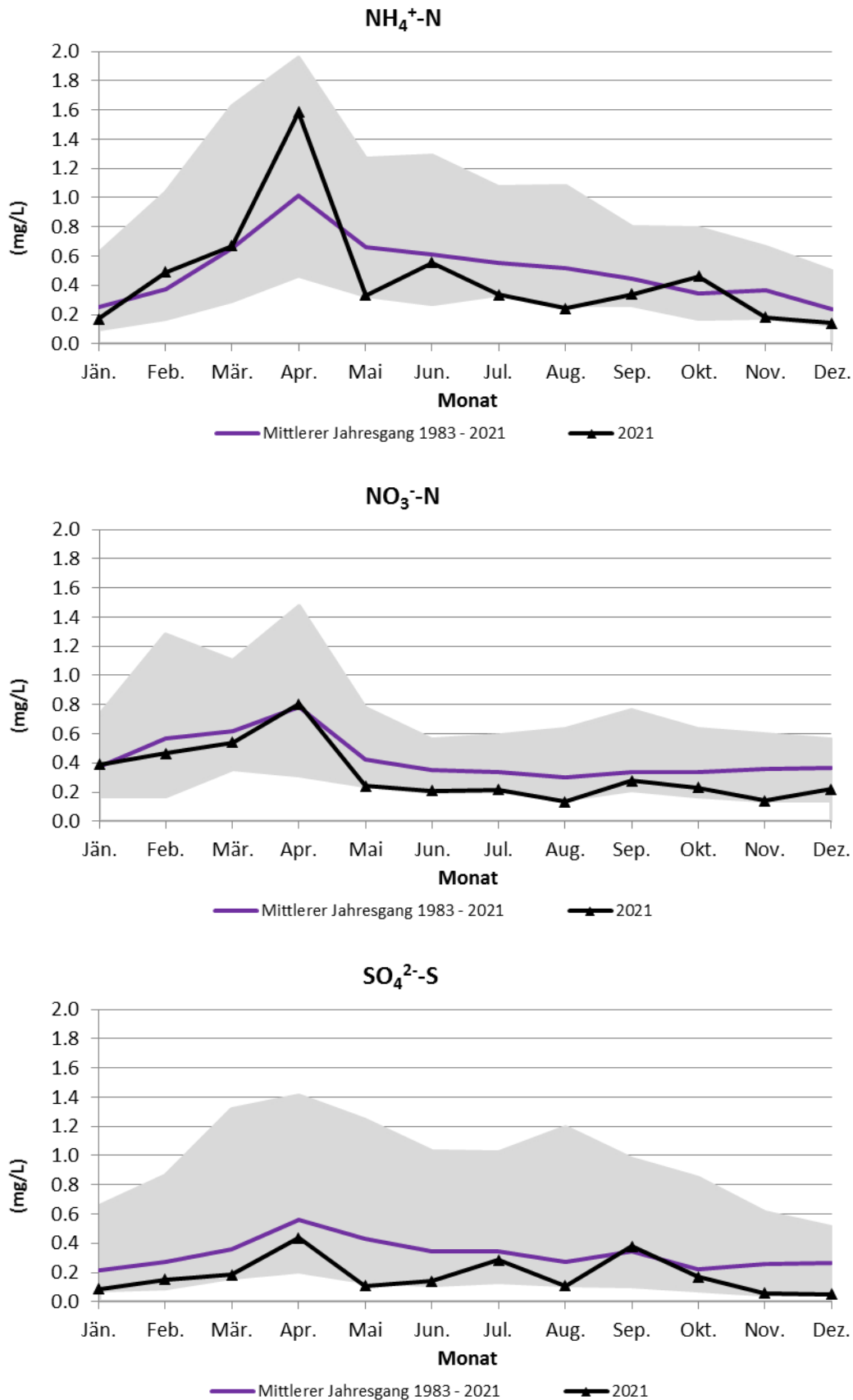
Abbildung. 10: Darstellung der mittleren monatlichen Konzentrationen in der Untersuchungsperiode 2021 im Vergleich zu den mittleren Jahresgängen an der Messstelle in Niederndorferberg . Die grau hinterlegte Fläche stellt die Schwankungsbreite der bisher bestimmten Monatswerte dar. Weitere Angaben im Text.
