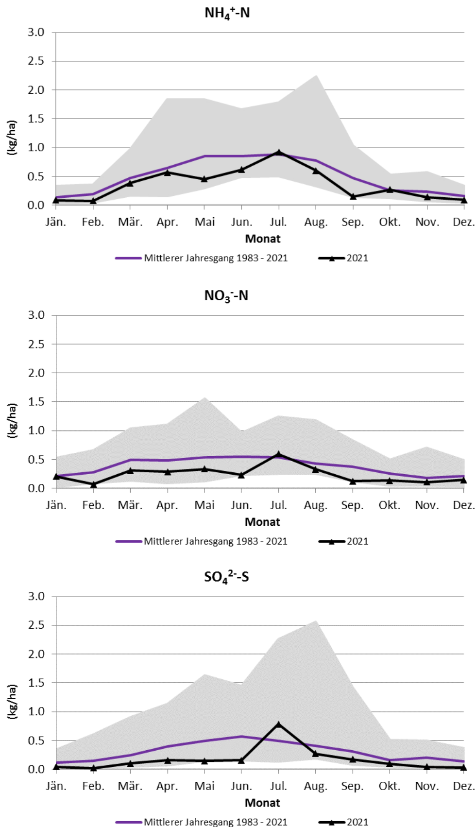
Abbildung 11: Darstellung der mittleren monatlichen Einträge in der Untersuchungsperiode 2021 im Vergleich zu den mittleren Jahresgängen an der Messstelle in Niederndorferberg . Die grau hinterlegte Fläche stellt die Schwankungsbreite der bisher bestimmten Monatswerte dar. Weitere Angaben im Text.
