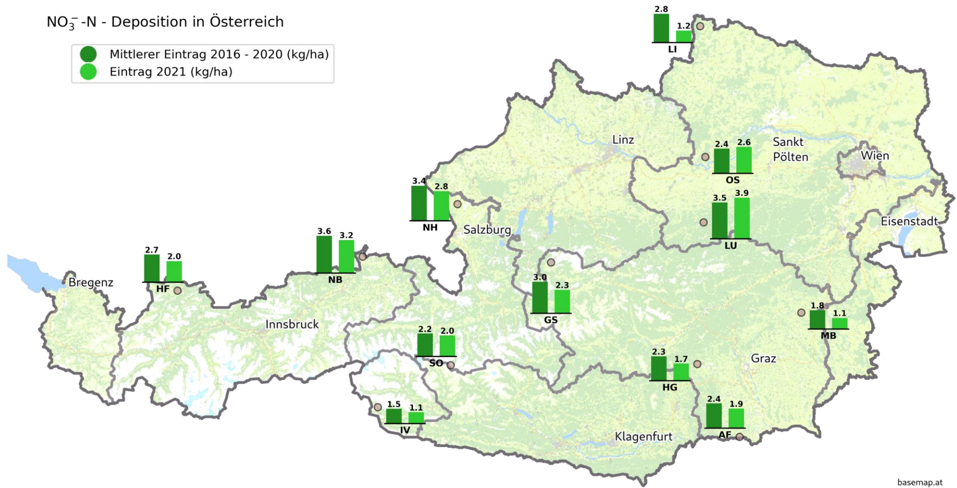
Abbildung 31: Räumliche Verteilung der NO 3 - -N-Jahreseinträge für den Zeitraum Jänner 2021 bis Dezember 2021 im Vergleich mit dem Mittelwert der letzten 5 Jahre.
