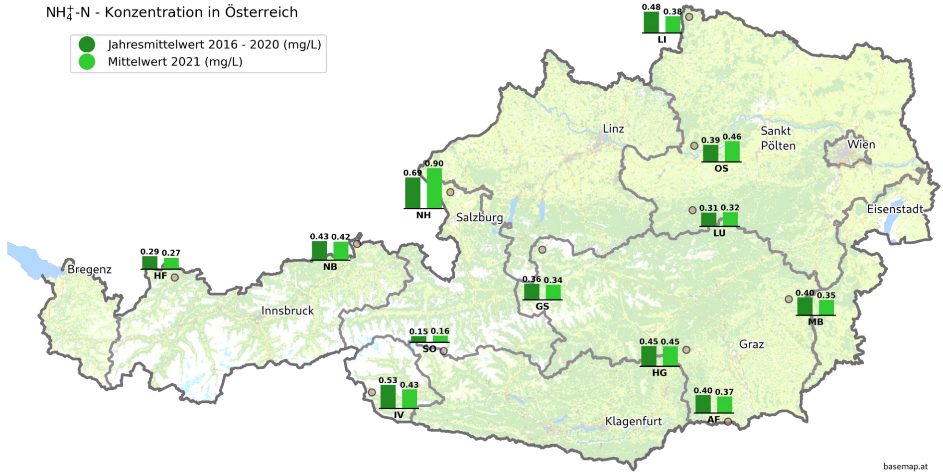
Abbildung 28: Räumliche Verteilung der mengengewichteten NH 4 + -N-Jahreskonzentrationen für den Zeitraum Jänner 2021 bis Dezember 2021 im Vergleich mit dem Mittelwert der letzten 5 Jahre.
