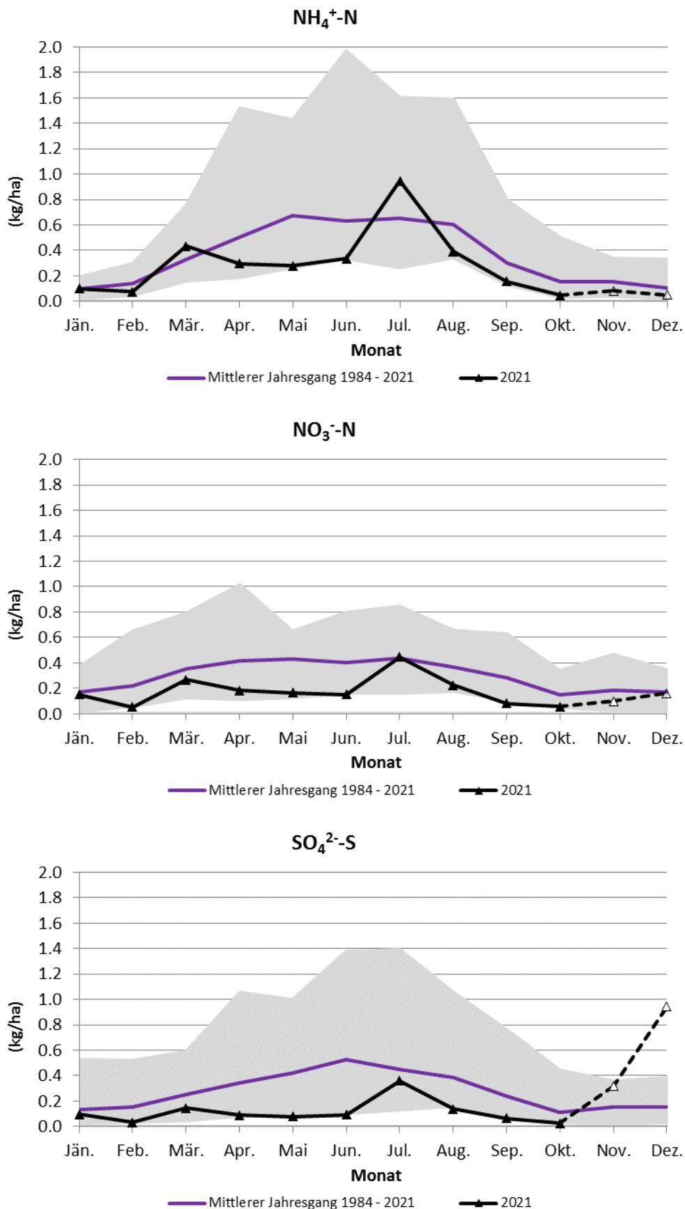
Abbildung 9: Darstellung der mittleren monatlichen Einträge in der Untersuchungsperiode 2021 im Vergleich zu den mittleren Jahresgängen an der Messstelle in Höfen . Die grau hinterlegte Fläche stellt die Schwankungsbreite der bisher bestimmten Monatswerte dar. Weitere Angaben im Text.
