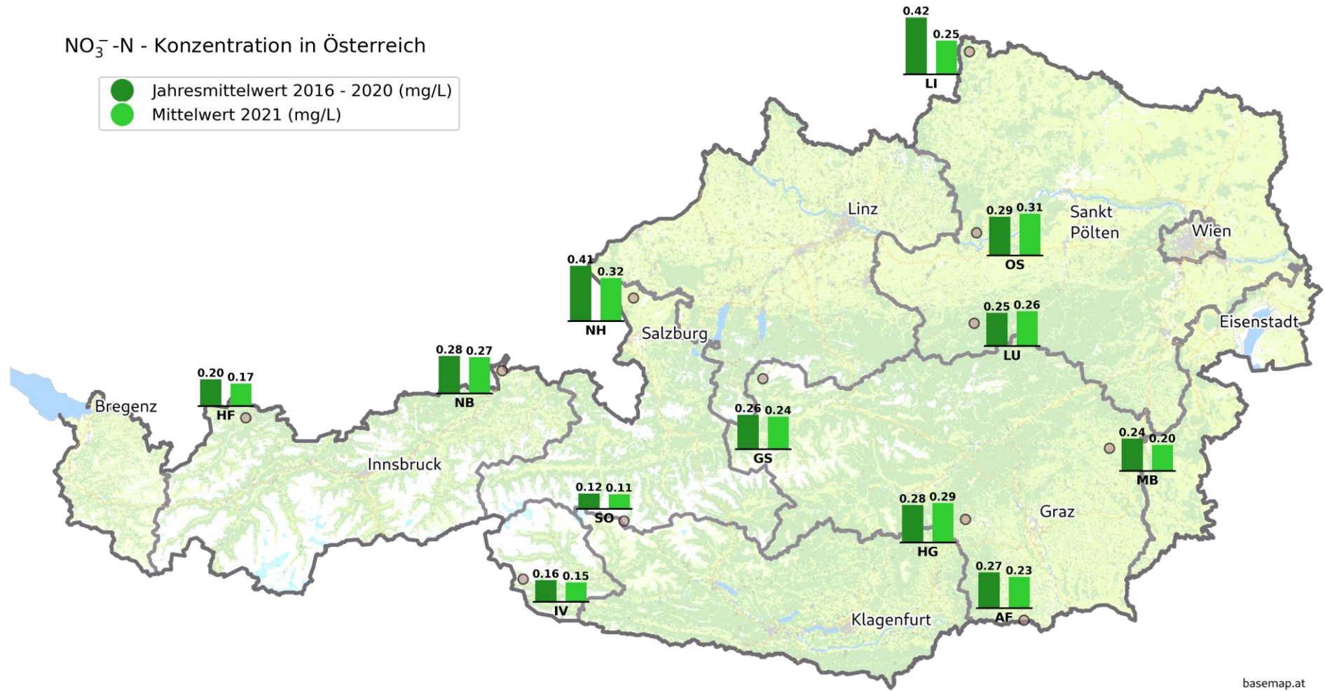
Abbildung 30: Räumliche Verteilung der mengengewichteten NO 3 - -N-Jahreskonzentrationen für den Zeitraum Jänner 2021 bis Dezember 2021 im Vergleich mit dem Mittelwert der letzten 5 Jahre.
