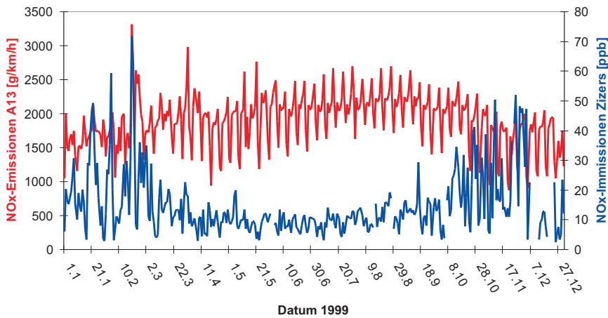
Vergleich NOx-Emissionen und -Immissionen
