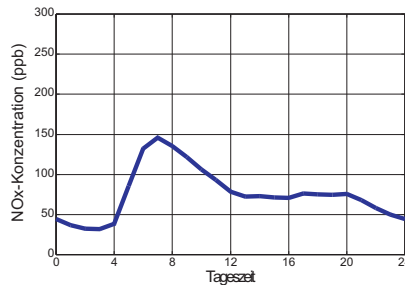
Mittlerer jährlicher Tagesgang
