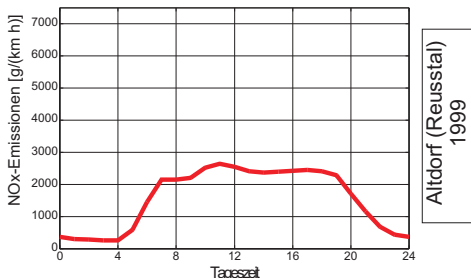
Mittlerer jährlicher Tagesgang
