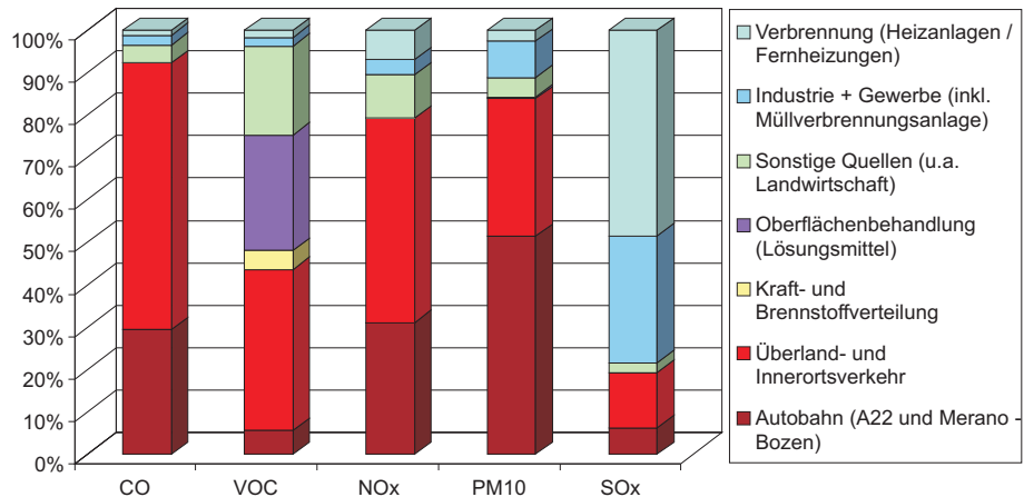
Emissionen nach Schadstoffquellen in Südtirol, Jahr 2000
