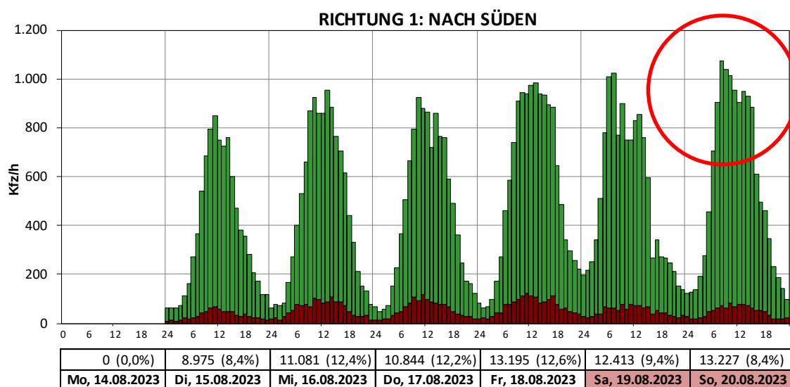
Abbildung 4-9: Wochenganglinie B179 Umfahrung Heiterwang, KW 33, Richtung
