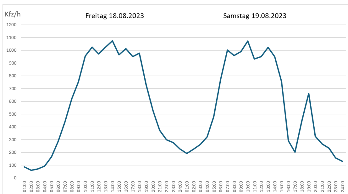
Abbildung 4-3: Tagesganglinie Zst 8826 Bichlbach, Fahrtrichtung Nassereith
