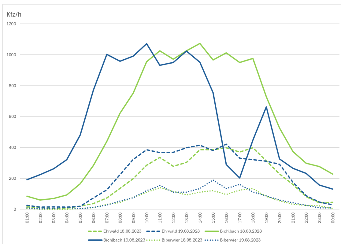
Abbildung 4-4: Tagesganglinien vom Freitag, den 18.08.2023 und Samstag, den 19.08.2023, Zst. Bichlbach, Ehrwald und Biberwier Fahrtrichtung Nassereith
