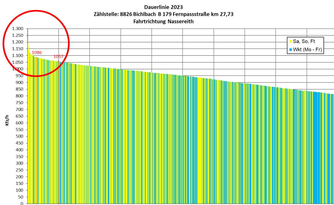
Abbildung 4-8: Dauerlinie der stündlichen Verkehrsstärken an der Zählstelle 8826 Bichlbach 2023
