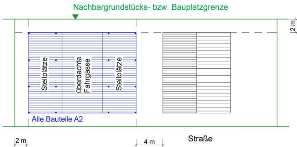
Abbildung 8: zu Punkt 4.2 – Überdachte Stellplätze > 250 m 2 mit überdachten Fahrgassen, freistehend
