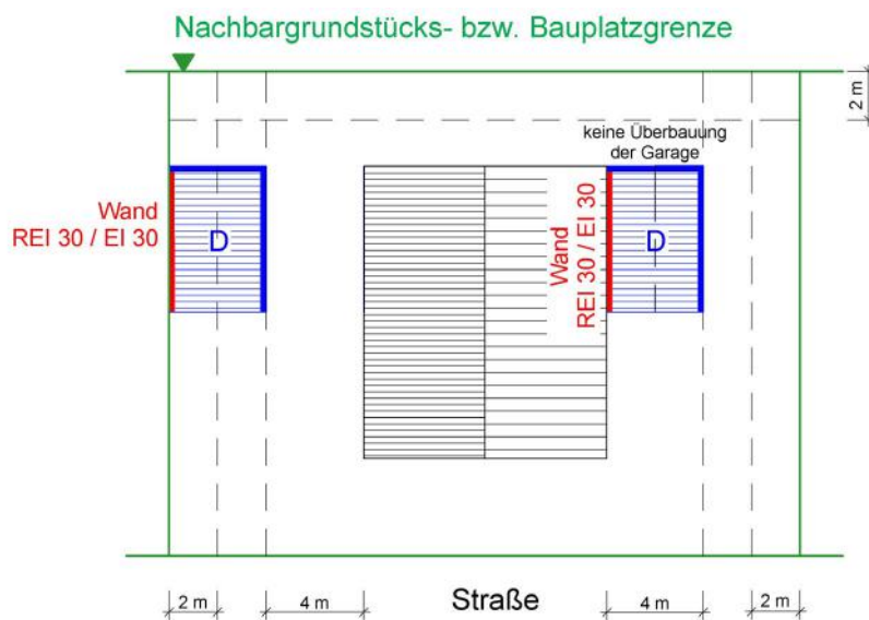
Abbildung 2: zu Punkt 2.2 – Garagen \leq 50 \text{ m}^2
