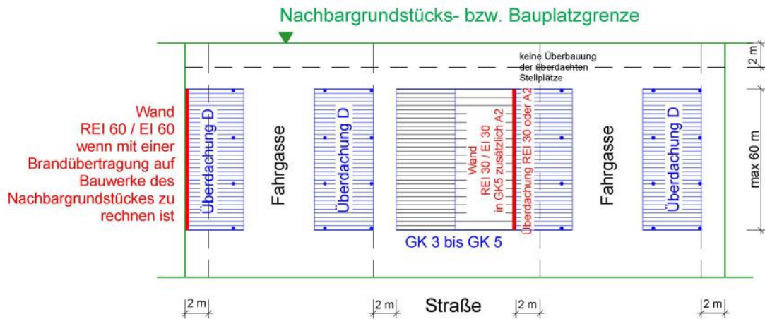
Abbildung 7: zu Punkt 4.1 – Überdachte Stellplätze > 250 m 2 ohne überdachte Fahrgassen bei Gebäuden der GK 3 bis GK 5
