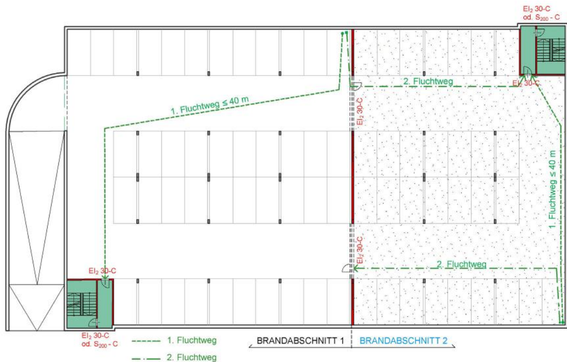
Abbildung 10: zu den Punkten 5.5.1 c) und 5.5.2 b) – Fluchtwege
