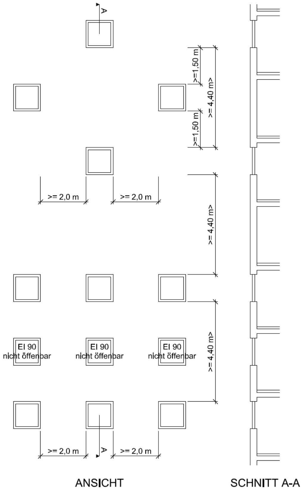
Abbildung 1: zu Punkt 3.4 d) – Maßnahmen zur wirksamen Einschränkung einer vertikalen Brandübertragung
