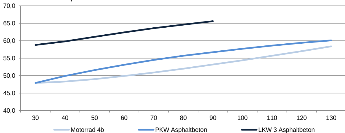
Abbildung 17: Emissionsverhalten als längenbezogener Schallleistungspegel für Motorrad, PKW und LKW pro Stunde
