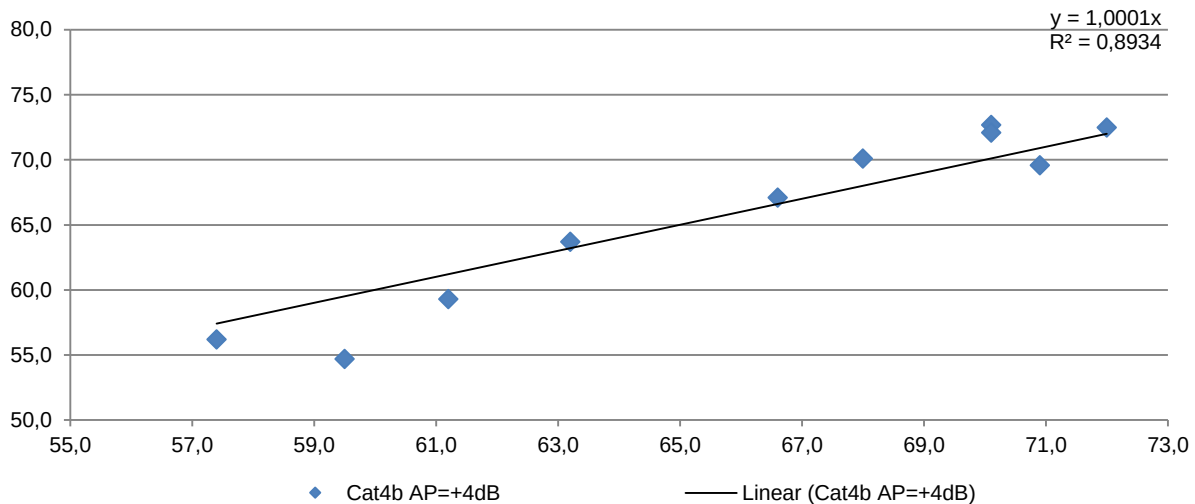
Abbildung 19: Zusammenhang der längenbezogenen Schallleistungspegel gemessen und berechnet mit +4 dB Anpassung
