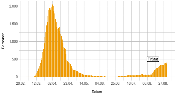
Aktiv Infizierte in Tirol
