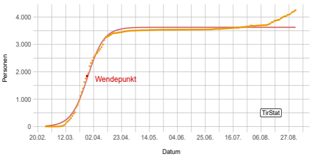
Positiv getestete Personen in Tirol (kumuliert) (rot = logistische Funktion)
