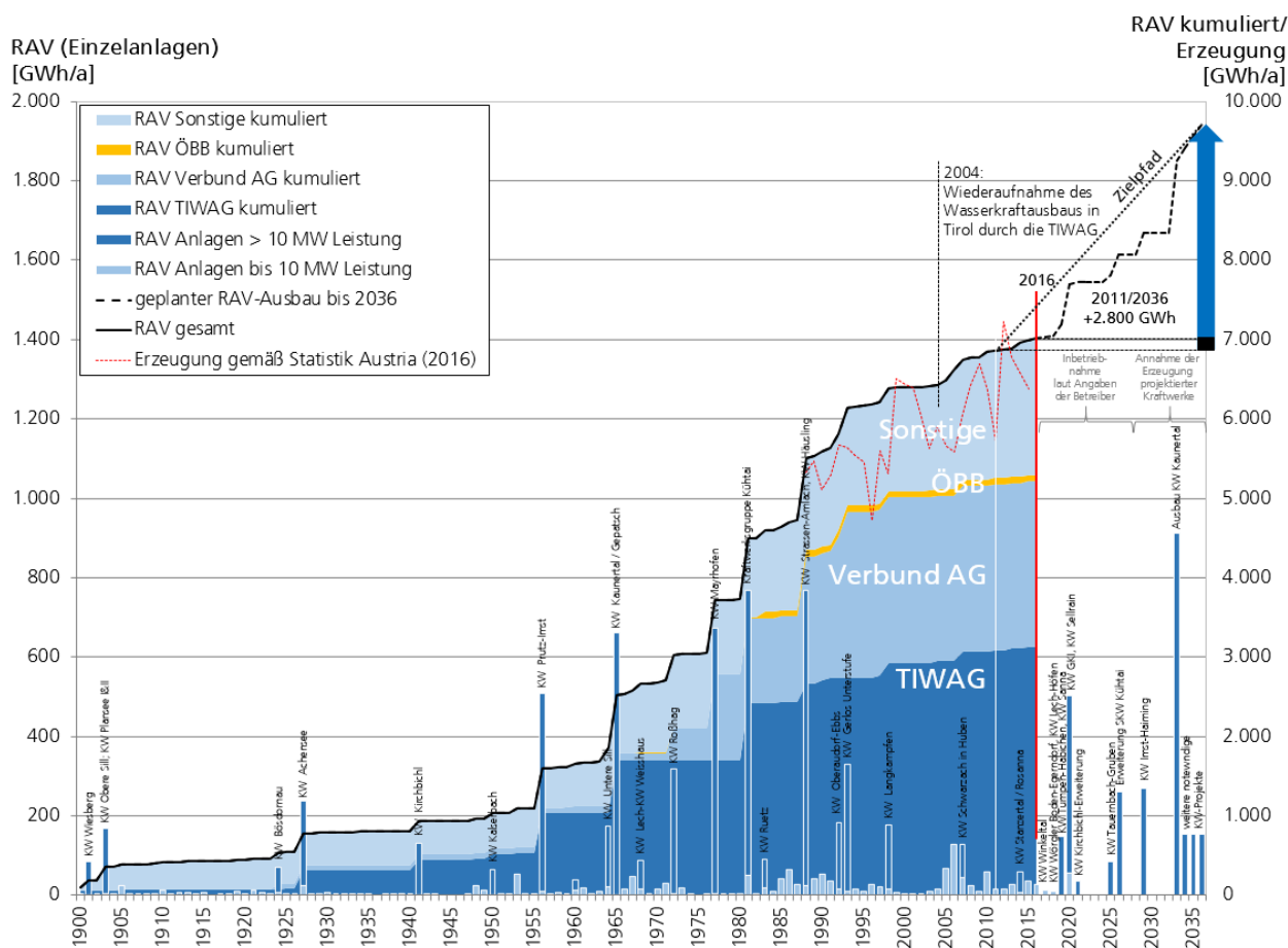
Abb. 3: Entwicklung des Tiroler Wasserkraftausbaus und Zielpfad bis zum Jahr 2036.
