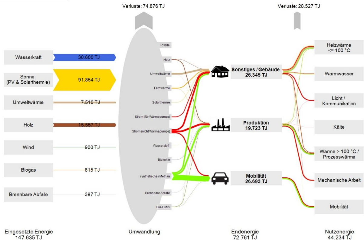
Abb. 19: Vereinfachte Darstellung der Energieflüsse 2050 Szenario III – „Methan-Szenario“.
