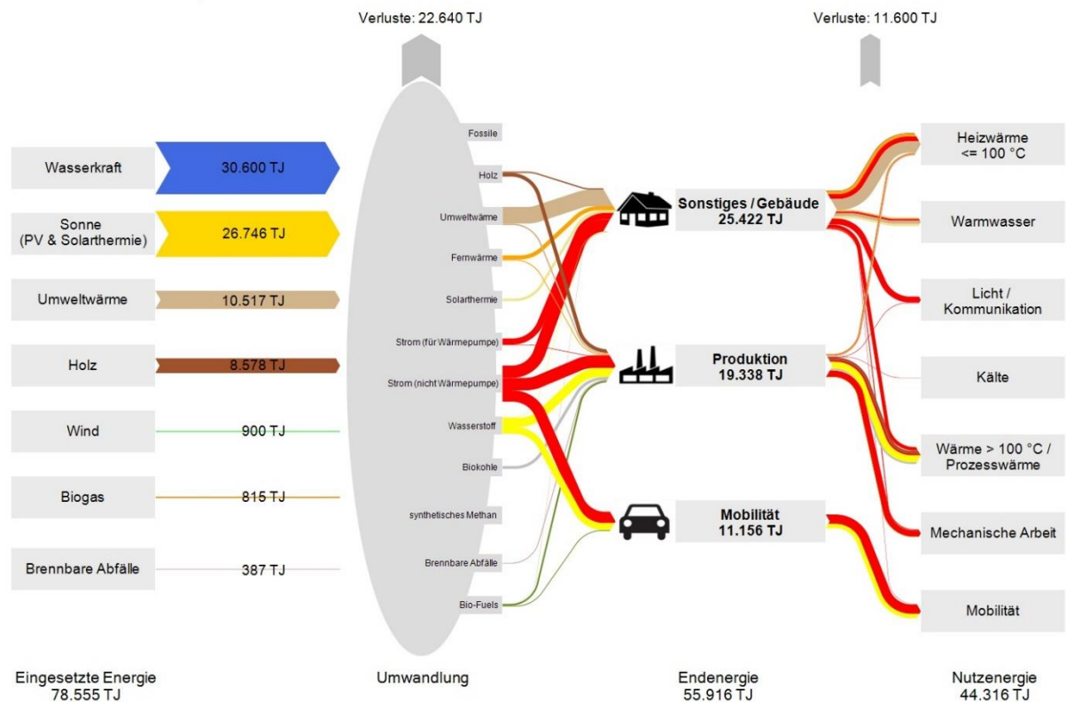
Abb. 18: Vereinfachte Darstellung der Energieflüsse 2050 Szenario II – „H 2 -Szenario“.
