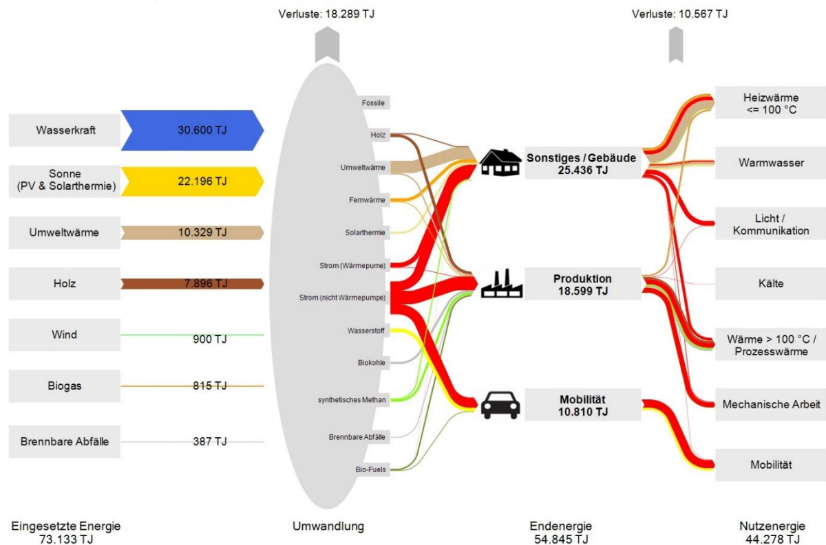
Abb. 21: Vereinfachte Darstellung der Energieflüsse Szenario IV – Szenario „Energienmix“.
