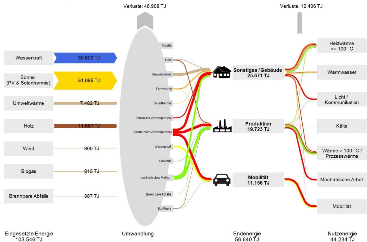
Abb. 20: Vereinfachte Darstellung der Energieflüsse Szenario IIIa – „adaptiertes Methan-Szenario“.
