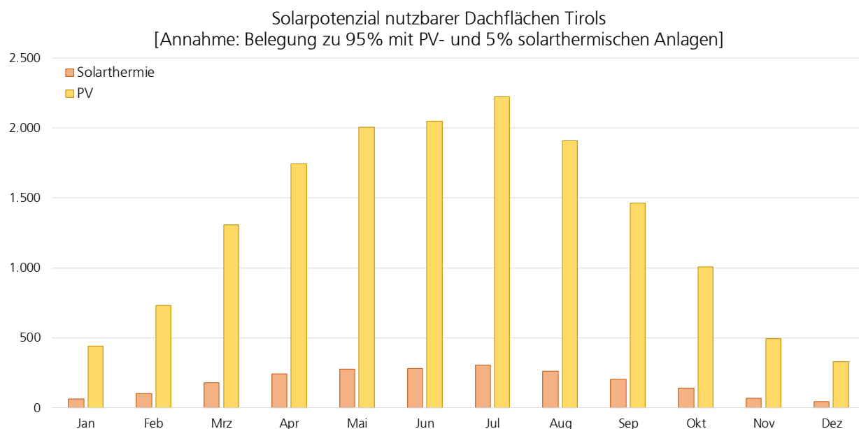
Abb. 6: Monatliche Erzeugungspotenziale von PV- und solarthermischen Anlagen bei Vollbelegung nutzbarer Dachflächen mit 95% PV- und 5% solarthermischen Anlagen.
