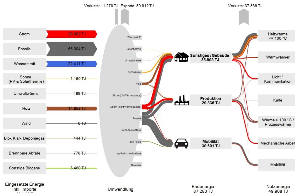
Abb. 14: Vereinfachte Darstellung der Energieflüsse in Tirol 2016.
