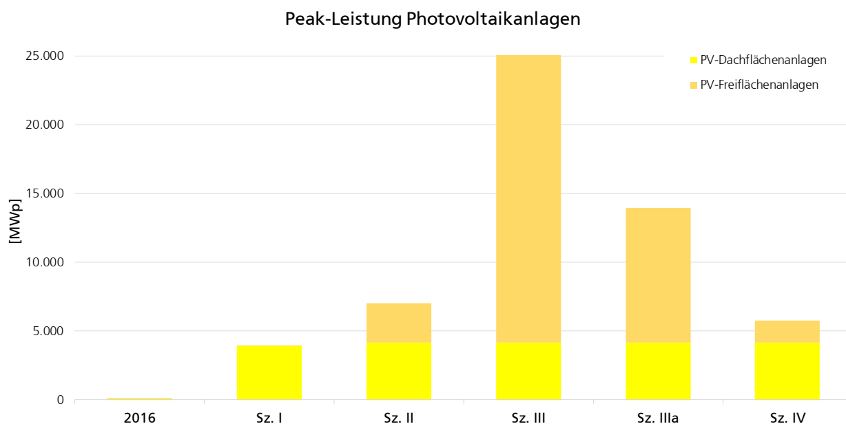
Abb. 23: MWp-Leistungen der notwendigen PV-Anlagen (Dach und Freifläche) der Szenarien.
