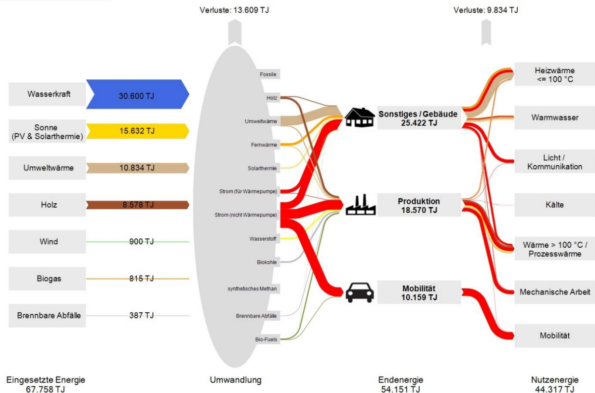
Abb. 17: Vereinfachte Darstellung der Energieflüsse 2050 im Szenario I – „Strom-Szenario“.
